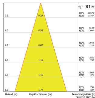
Kegeldiagramm | FL 34,0°
